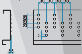
フロア材(エンボス加工)拡大図
