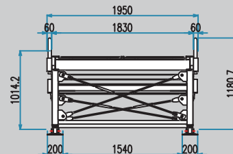
スロープ A矢視図
